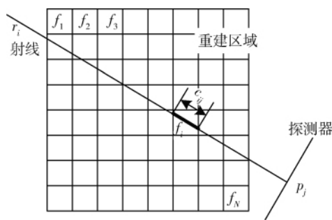
(a) 长度权值法
