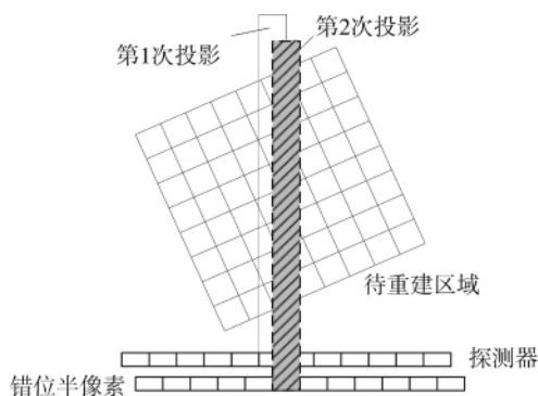
图 1 半像素错位法采样示意图
