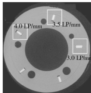
图 9 CT 重建图像
