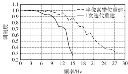
图 7 面积权值重建算法 MTF 曲线
