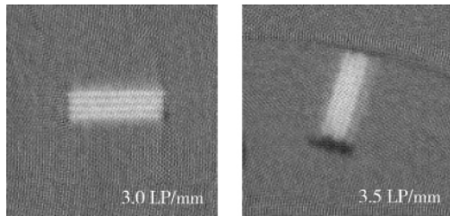
(a) 标准扫描长度权值直接重建法
