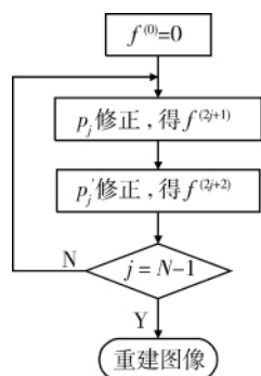
图2 直接重建算法流程图
